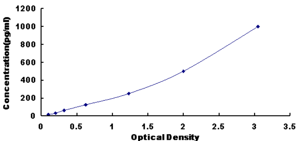
图 1: 人成纤维细胞生长因子 3(FGF3)试剂盒标准曲线
