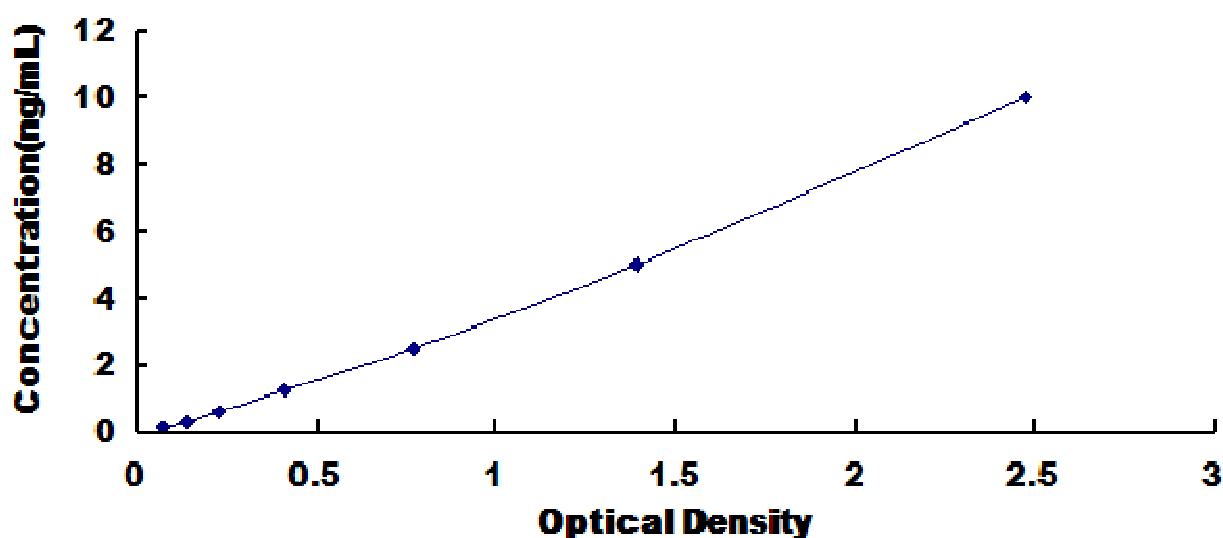
人成纤维细胞生长因子受体 1 (FGFR1) 试剂盒标准曲线
