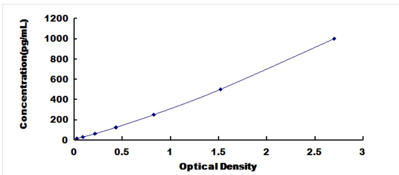
人含Ⅲ型纤连蛋白域蛋白 5 (FNDC5) 检测试剂盒标准曲线
