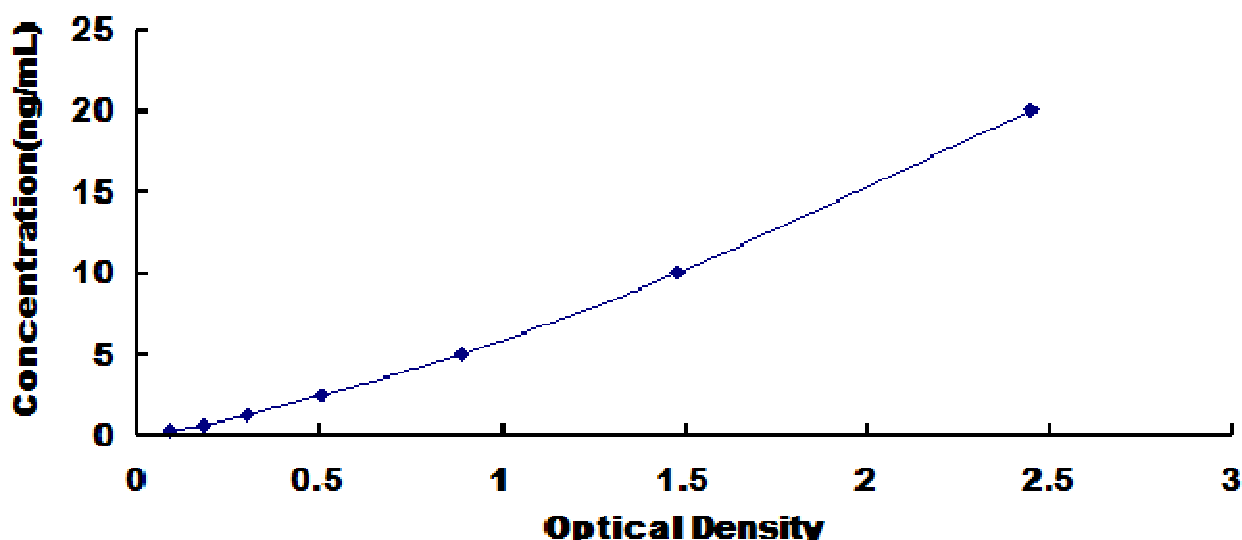
人纤维胶凝蛋白 3 (FCN3) 检测试剂盒标准曲线
