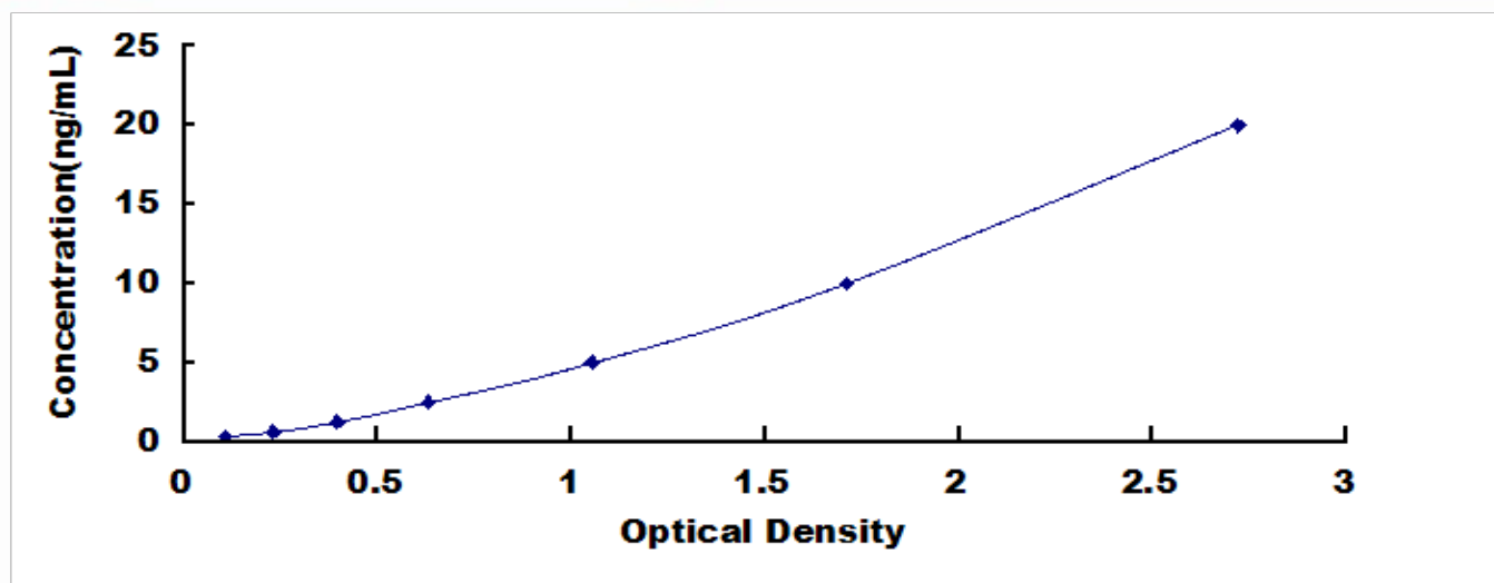
人丝蛋白 C \gamma (FLNC) 检测试剂盒标准曲线
