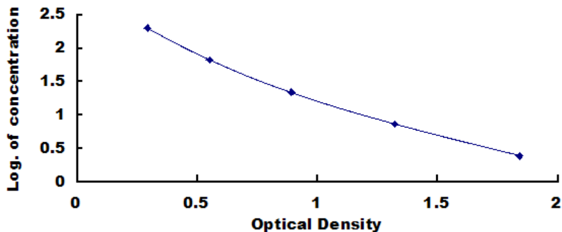
犬促卵泡素 (FSH) 检测试剂盒标准曲线
