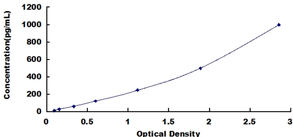
人岩藻糖苷酶 \alpha L2 (FUC \alpha 2) 检测试剂盒标准曲线
