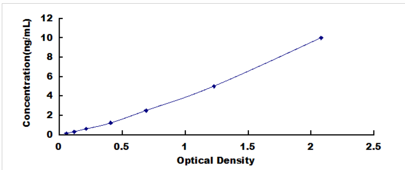
人融合蛋白 (FUS) 检测试剂盒标准曲线
