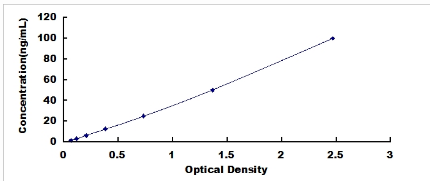
人半乳糖苷酶 \alpha (GL \alpha ) 检测试剂盒标准曲线
