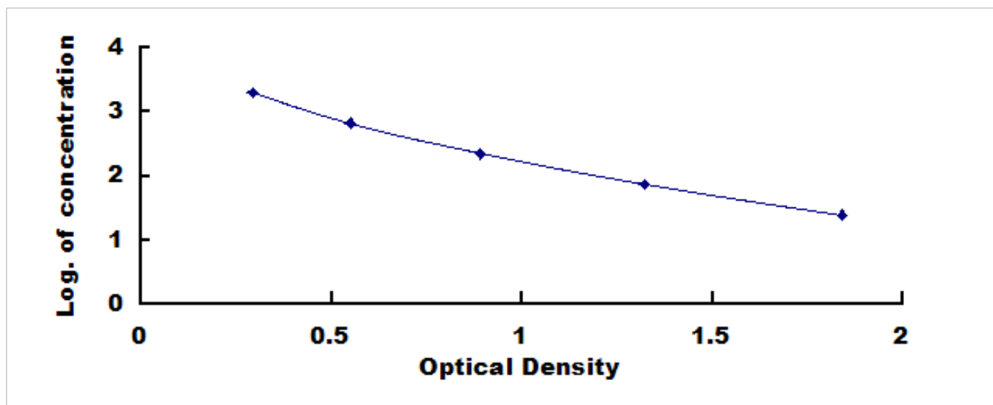
γ-氨基丁酸 (γ ABA) 检测试剂盒标准曲线
