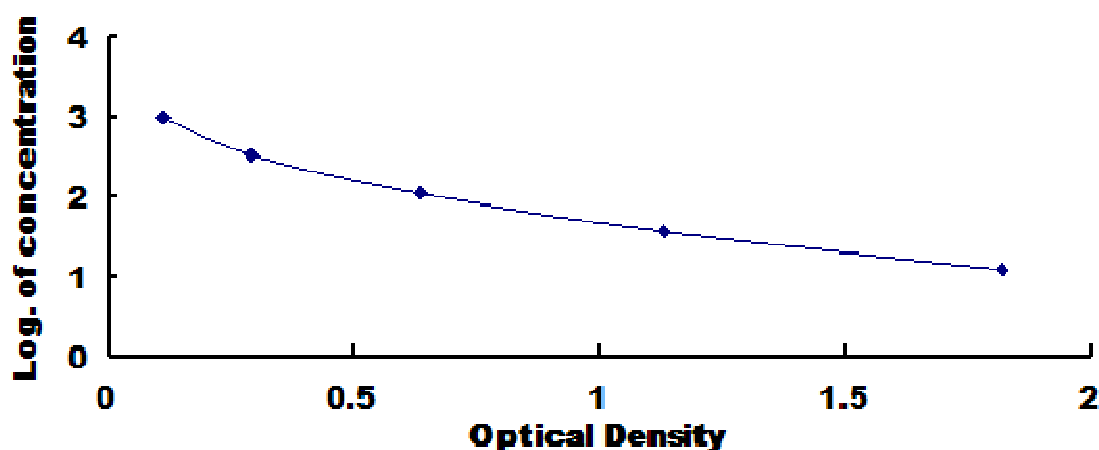
人胃泌素(GT)试剂盒标准曲线
