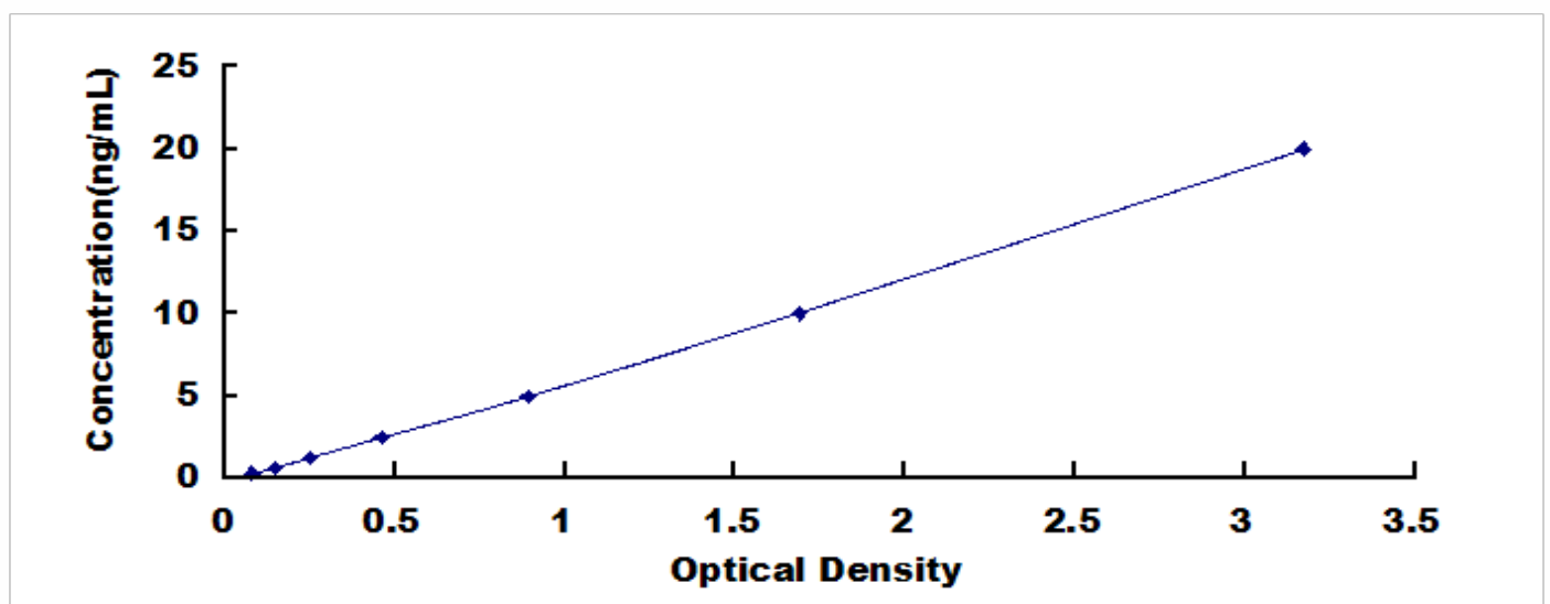
大鼠谷氨酸脱氢酶(GDH)检测试剂盒标准曲线
