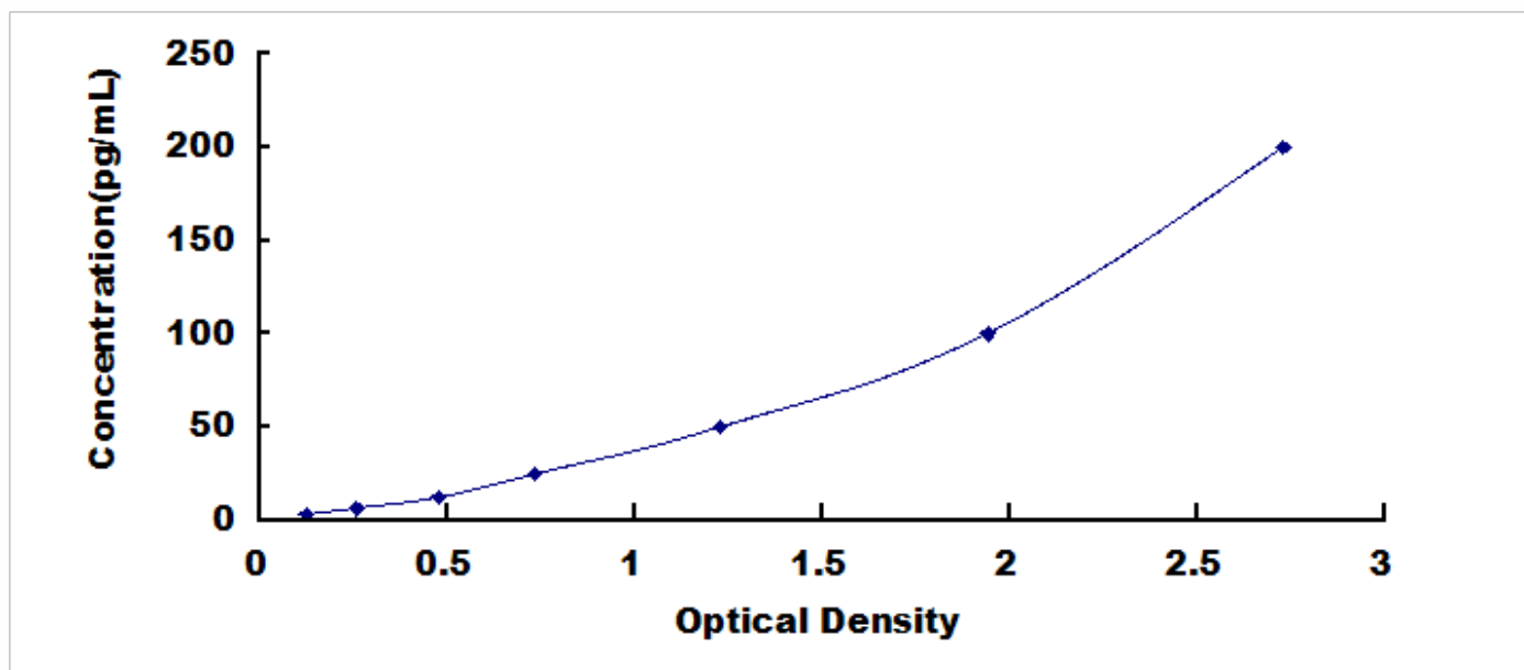
小鼠谷氨酰胺合成酶(GS)检测试剂盒标准曲线
