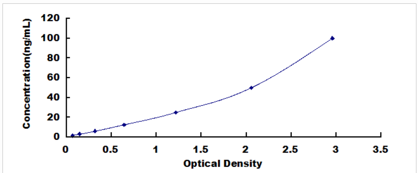
人血浆谷胱甘肽过氧化物酶(GPX3)检测试剂盒标准曲线
