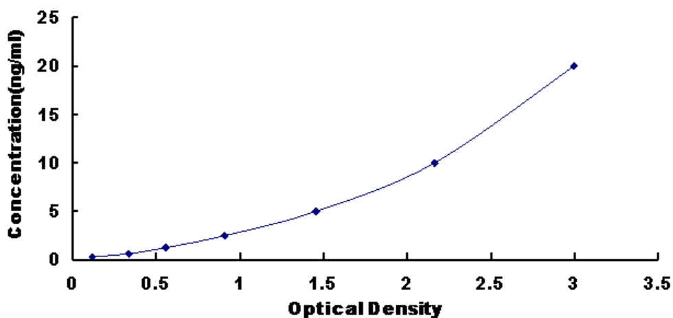
图 1: 人的谷胱甘肽 S 转移酶 \alpha 4(GST \alpha 4)试剂盒标准曲线
