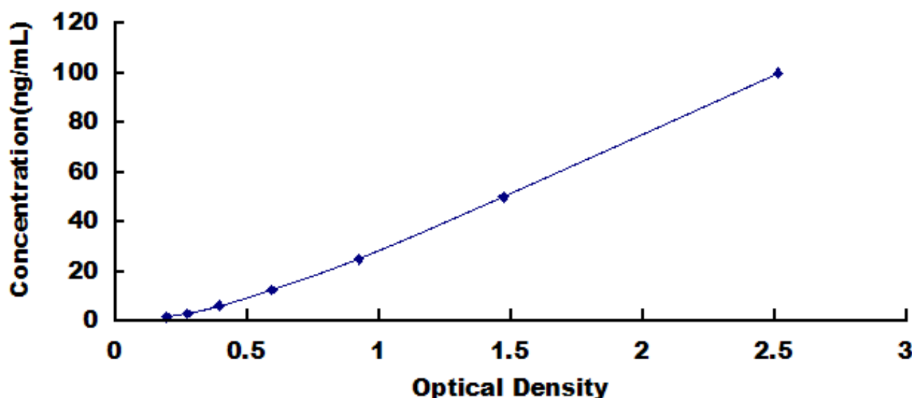
人谷胱甘肽 S 转移酶 \mu 1 (GST \mu 1) 试剂盒标准曲线
