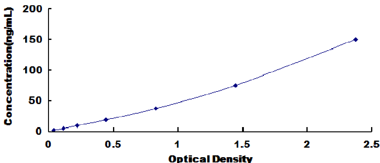
人谷胱甘肽 S 转移酶 \pi 1 (GST \pi 1) 检测试剂盒标准曲线
