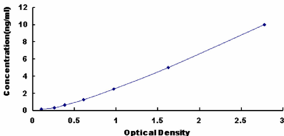
图 1：大鼠线粒体甘油 3 磷酸酰基转移酶(GPAM)试剂盒标准曲线
