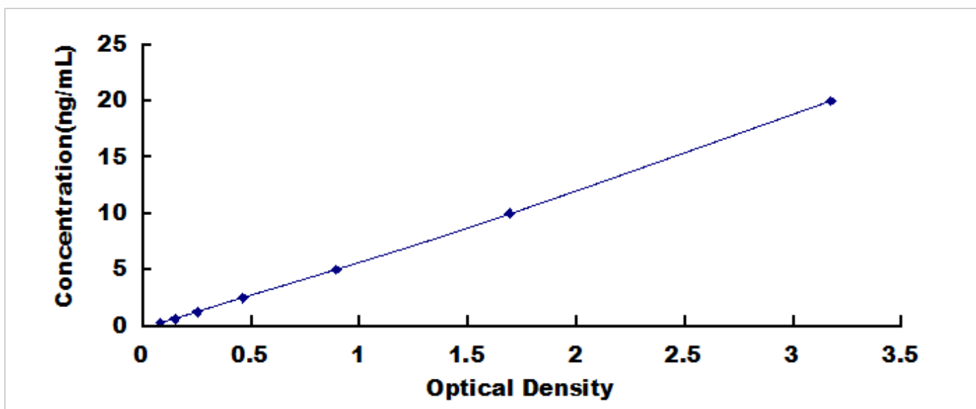
大鼠甘氨酸受体 \alpha 2 (GLR \alpha 2 ) 检测试剂盒标准曲线
