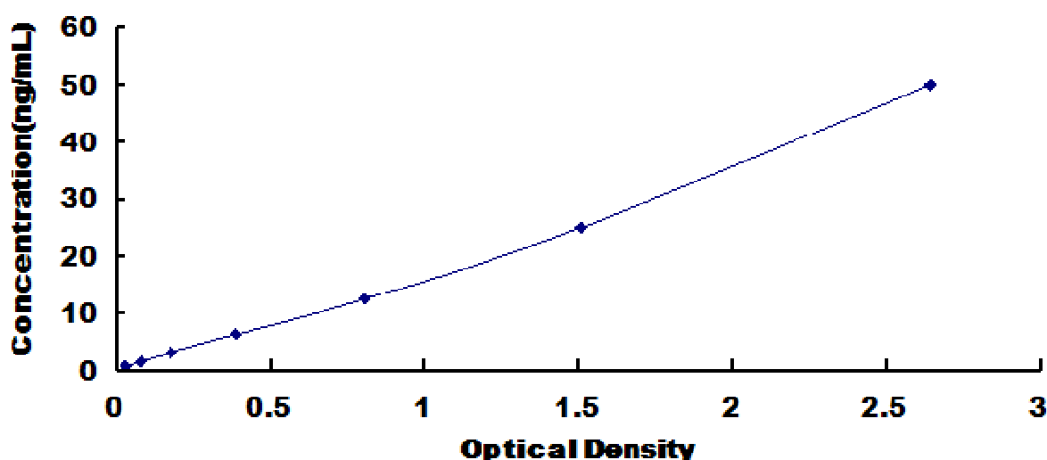
人糖基化磷脂酰肌醇特异性磷脂酶 D1 (GPLD1) 检测试剂盒标准曲线
