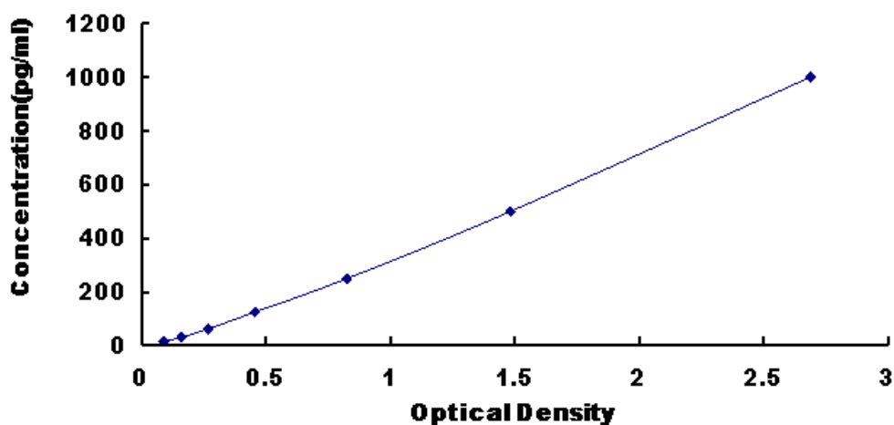
图 1: 人的促性腺激素释放激素(GnRH)试剂盒标准曲线
