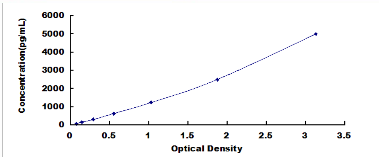
人生长分化因子 5 (GDF5) 检测试剂盒标准曲线
