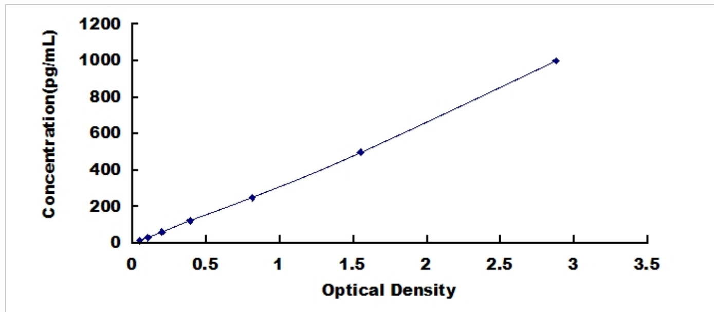
人生长分化因子 9 (GDF9) 检测试剂盒标准曲线
