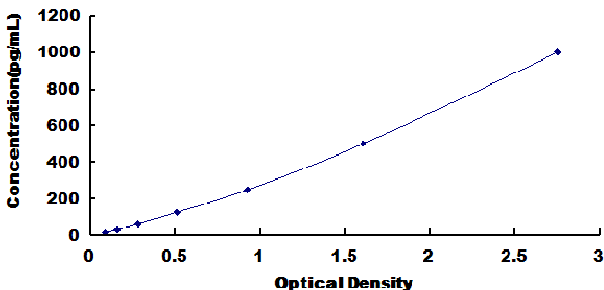
小鼠生长激素(GH)试剂盒标准曲线
