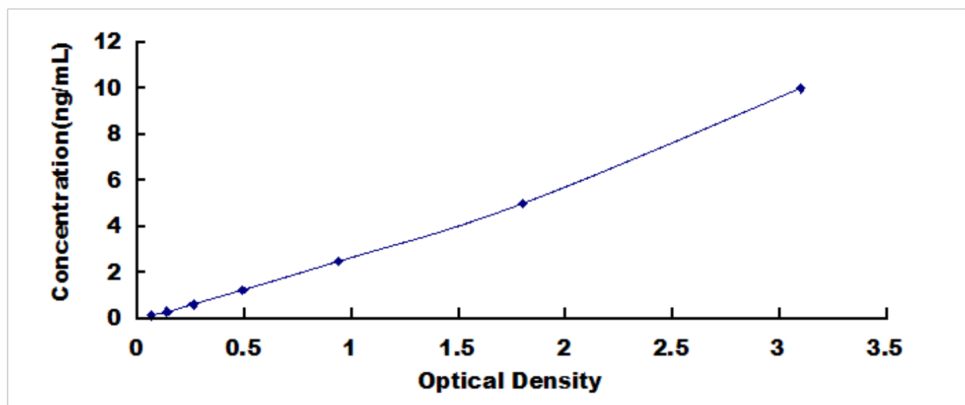
人 60kD 热休克蛋白 (HSPD1) 检测试剂盒标准曲线
