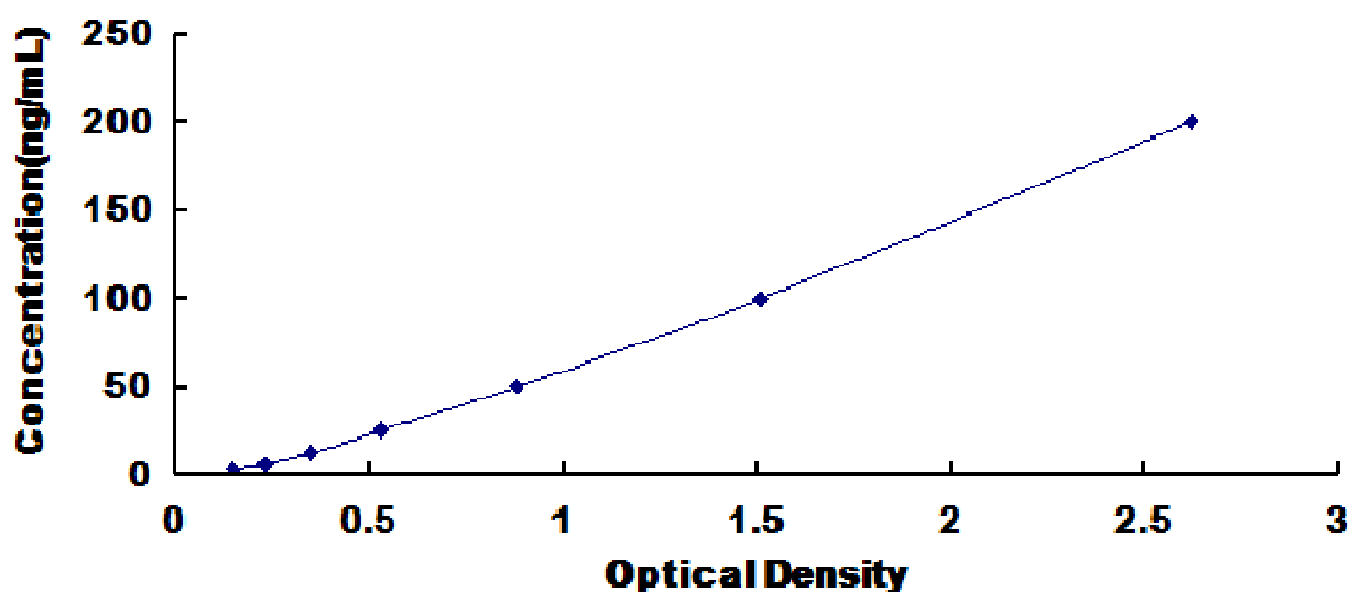
人热休克蛋白 70 (HSP70) 检测试剂盒标准曲线
