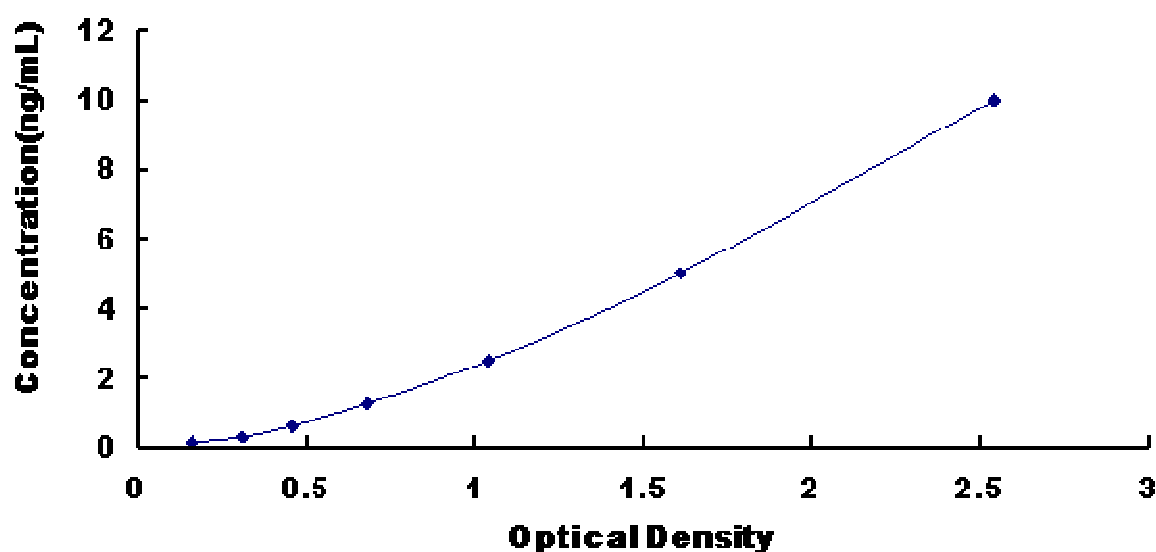
小鼠 Hedgehog 相互作用蛋白(HHIP)试剂盒标准曲线
