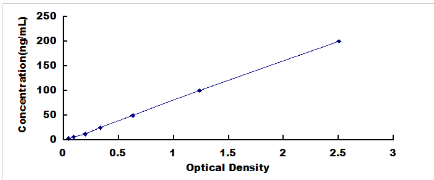
牛血红蛋白 (HB) 检测试剂盒标准曲线
