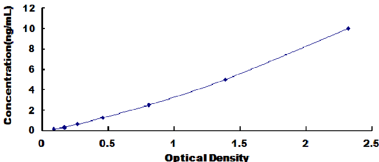
人血幼素(HJV)检测试剂盒标准曲线
