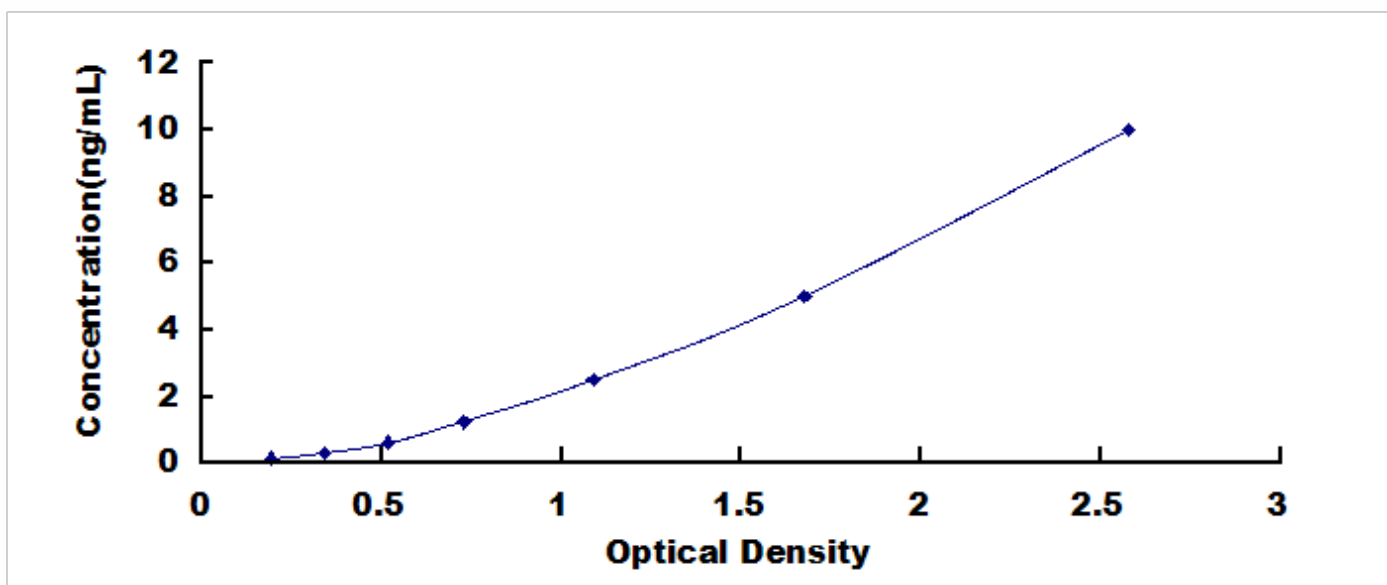
人硫酸肝素-6-O-磺基转移酶 2 (HS6ST2) 检测试剂盒标准曲线
