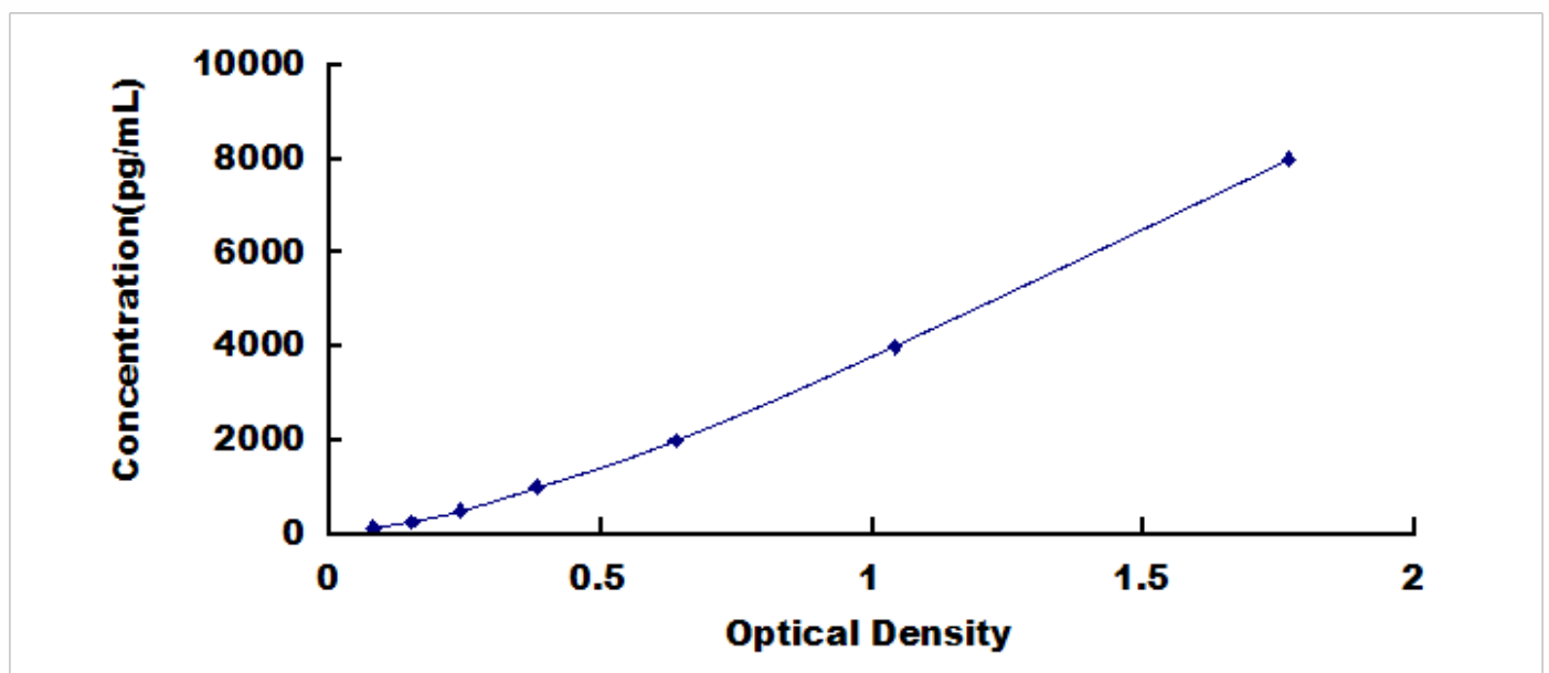
人硫酸肝素蛋白聚糖 2 (HSPG2) 检测试剂盒标准曲线
