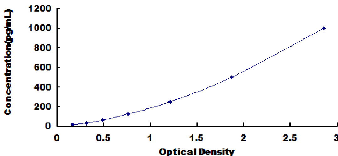
兔肝细胞生长因子(HGF)检测试剂盒标准曲线
