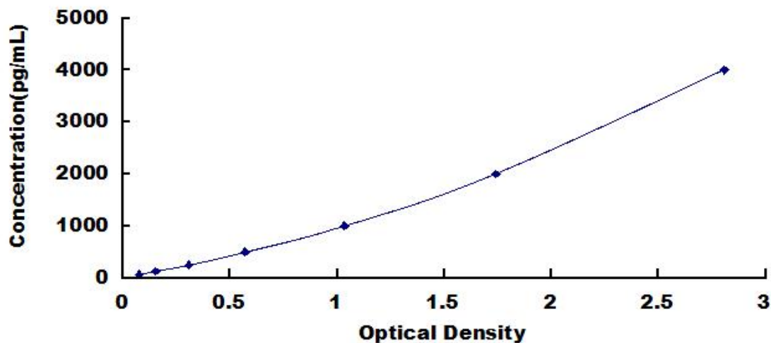
人高迁移率族蛋白 1 (HMG1) 检测试剂盒标准曲线
