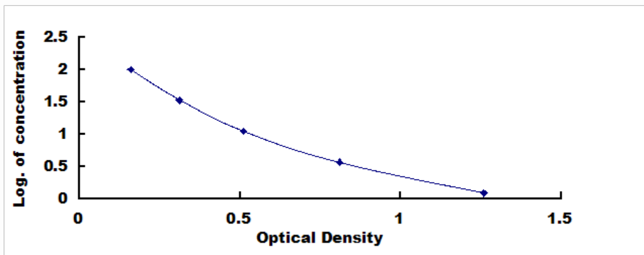
组胺(HA)检测试剂盒标准曲线
