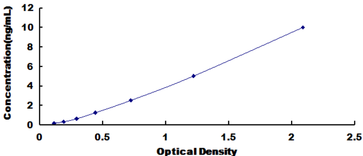
小鼠组蛋白 H4 (H4) 检测试剂盒标准曲线
