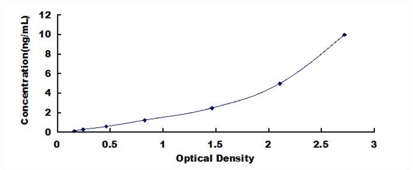
组蛋白 H4 (H4) 检测试剂盒标准曲线
