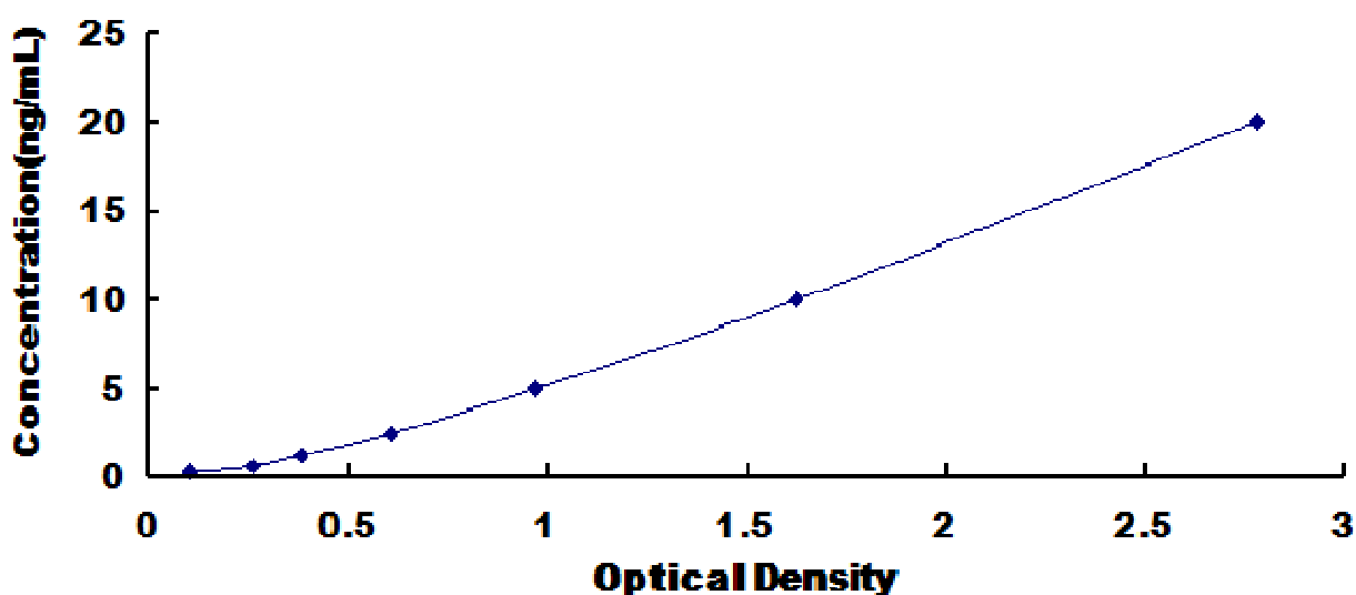
鸡免疫球蛋白 A(IgA) 检测试剂盒标准曲线
