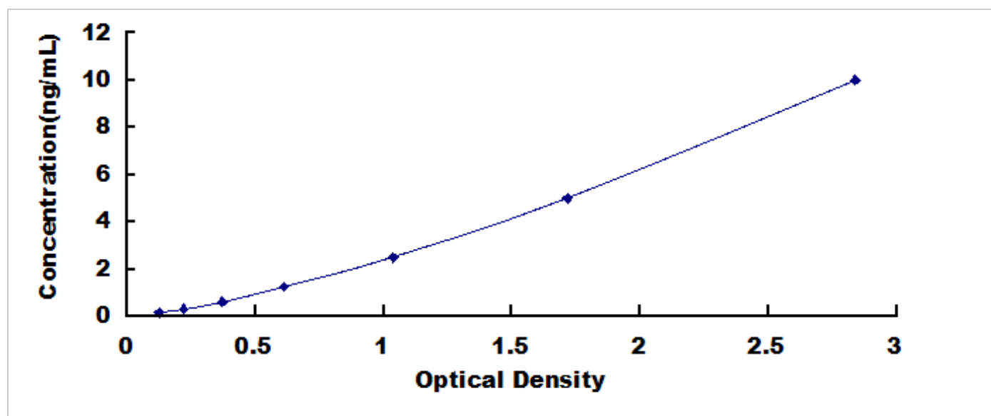
人免疫球蛋白 \kappa (Ig \kappa ) 检测试剂盒标准曲线
