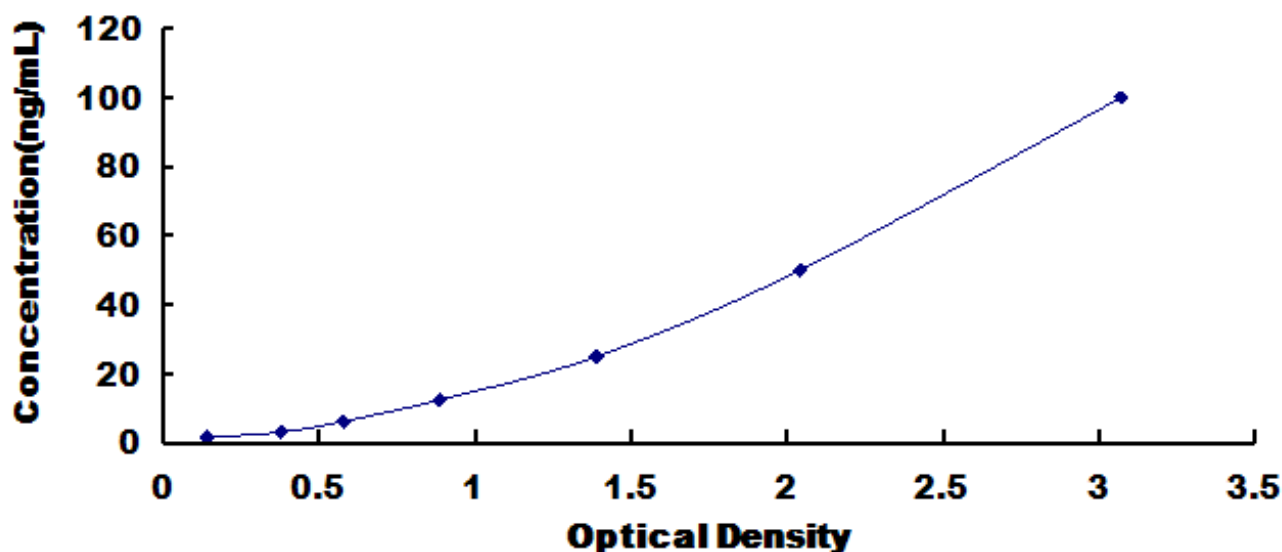
鸡免疫球蛋白 M(IgM) 检测试剂盒标准曲线
