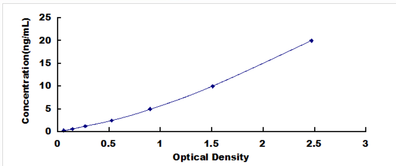
人吲哚胺 2,3-双加氧酶(IDO)检测试剂盒标准曲线
