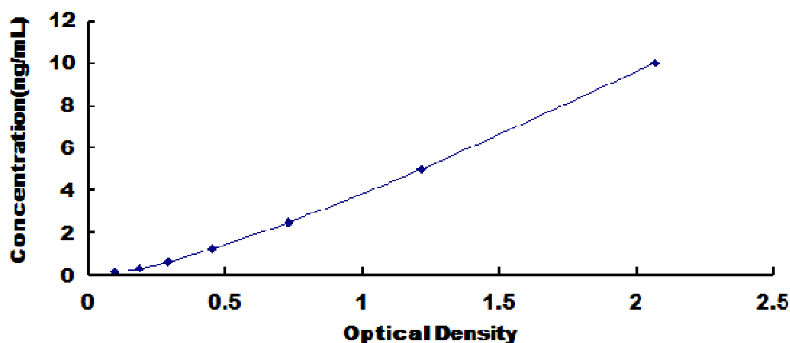
人核因子 \kappa B 抑制蛋白 \alpha (I \kappa B \alpha ) 试剂盒标准曲线
