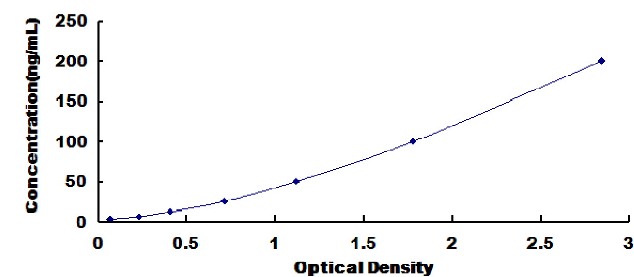
人胰岛素自身抗体(IAA)检测试剂盒标准曲线
