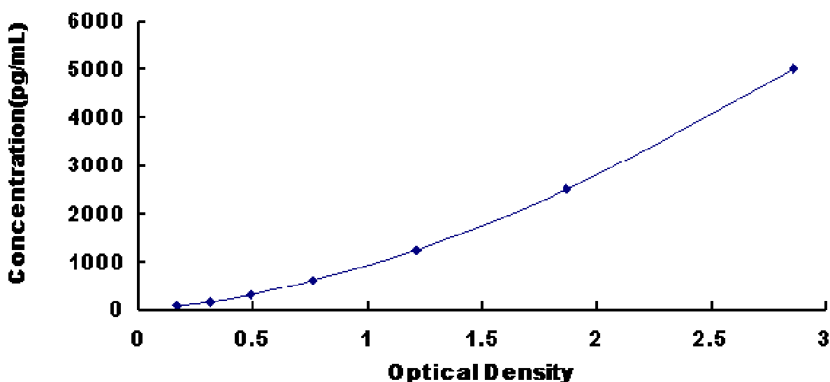
小鼠胰岛素降解酶(IDE)试剂盒标准曲线
