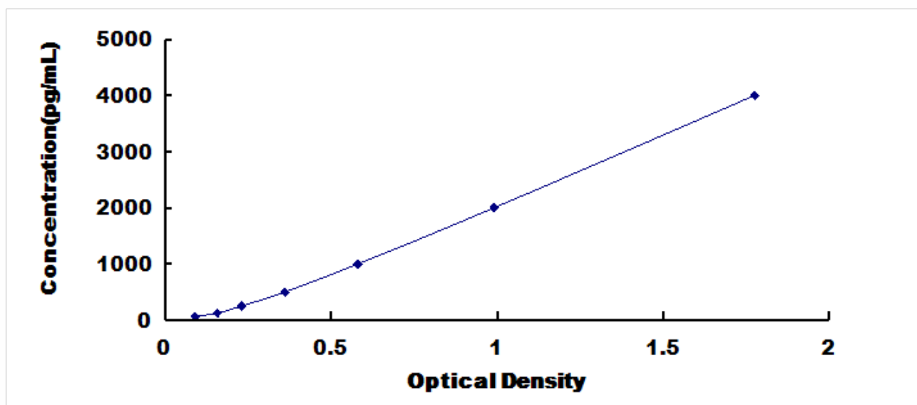
牛胰岛素样生长因子 1 (IGF1) 检测试剂盒标准曲线
