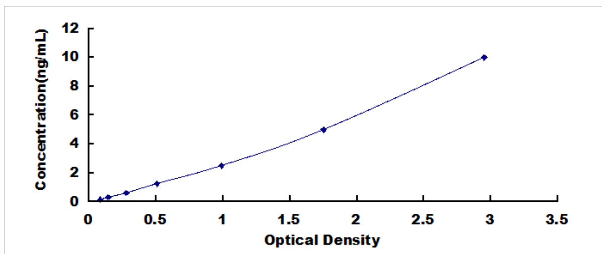
人胰岛素样生长因子 2-mRNA 结合蛋白 3 (IGF2BP3) 检测试剂盒标准曲线
