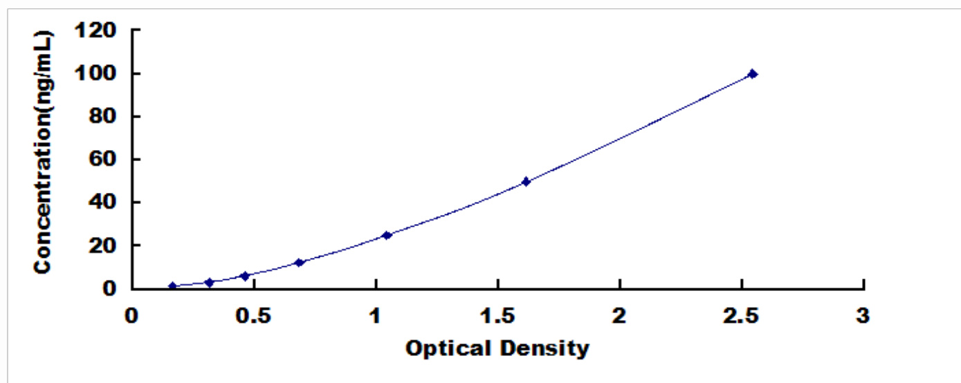
人胰岛素样生长因子酸不稳定亚基(IGFALS)检测试剂盒标准曲线
