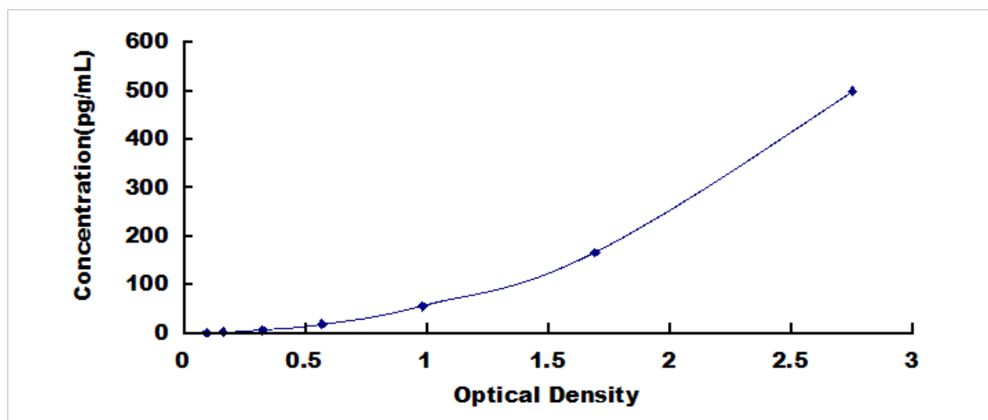
大鼠内凝集蛋白 1 (ITLN1) 检测试剂盒标准曲线
