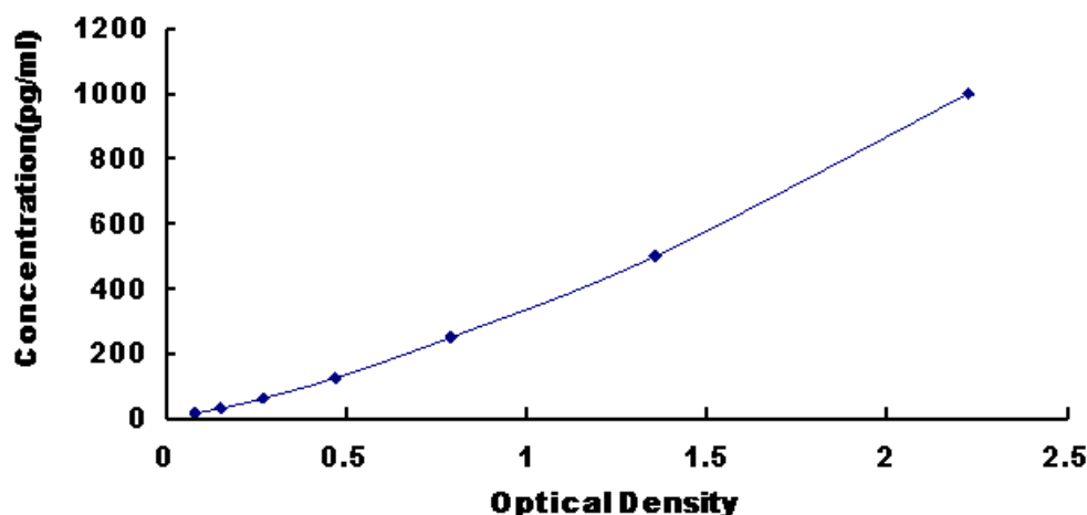
图 1: 豚鼠 \alpha 干扰素(IFN \alpha )试剂盒标准曲线
