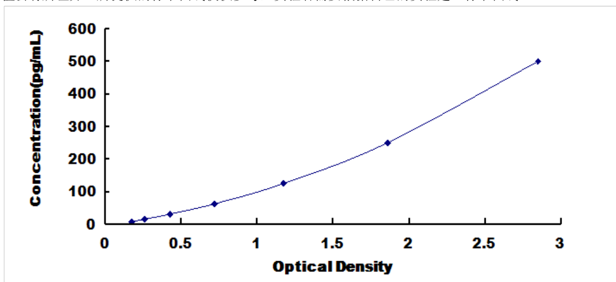
人干扰素 \alpha (IFN \alpha ) 检测试剂盒标准曲线
