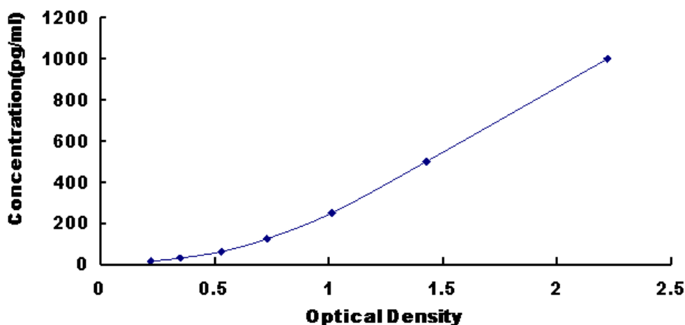
图 1: 兔的 \alpha 干扰素(IFN \alpha )试剂盒标准曲线
